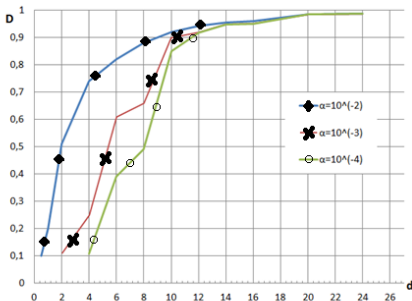
Рис. 2. Зависимость вероятности правильного обнаружения от соотношения сигнал/шум при заданных \alpha
