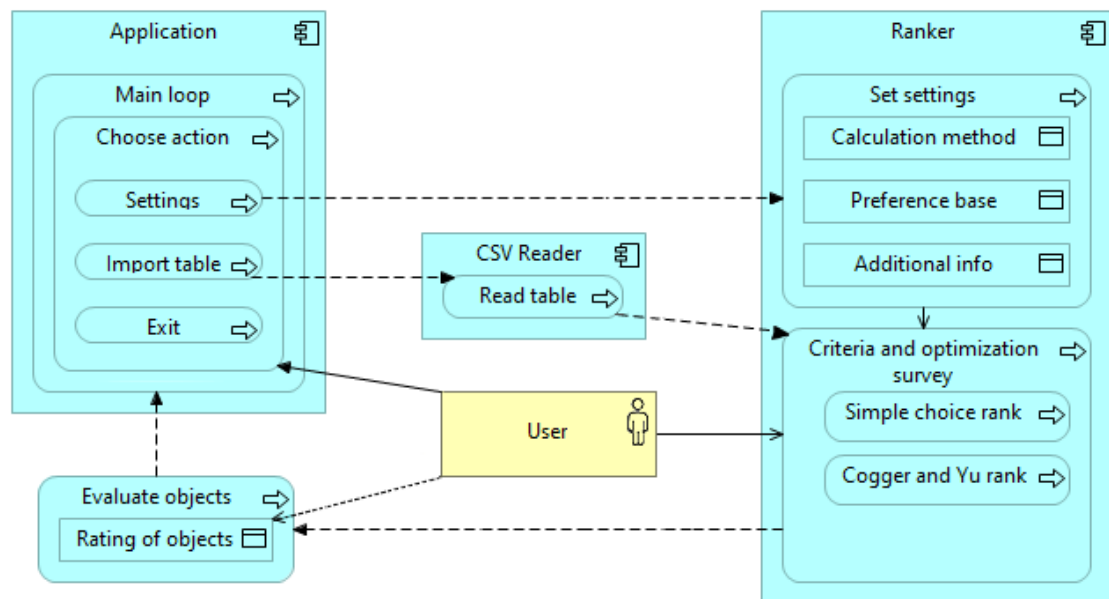
Рис. 1. Схема работы программы с реализацией метода Коггера и Ю
