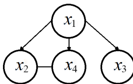
Рис. 3. Частичная упорядоченность вариантов по двум равноважным признакам [17]
