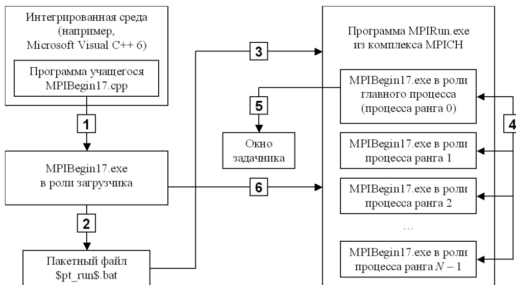
Рис. 1. Механизм выполнения задания в параллельном режиме:
