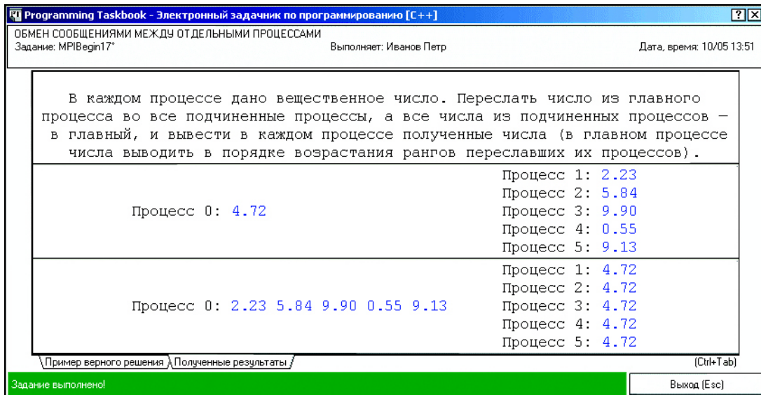
Рис. 2. Вид окна задачника Programming Taskbook при успешном выполнении задания MPIBegin17
